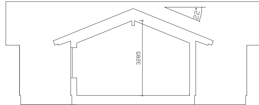
SEKTION B-B
